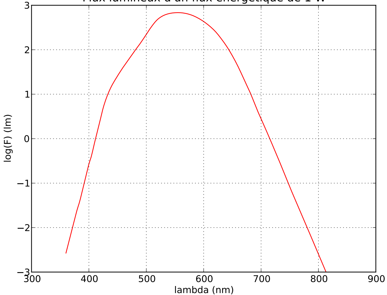
Flux lumineux d'un flux énergétique de 1 W
