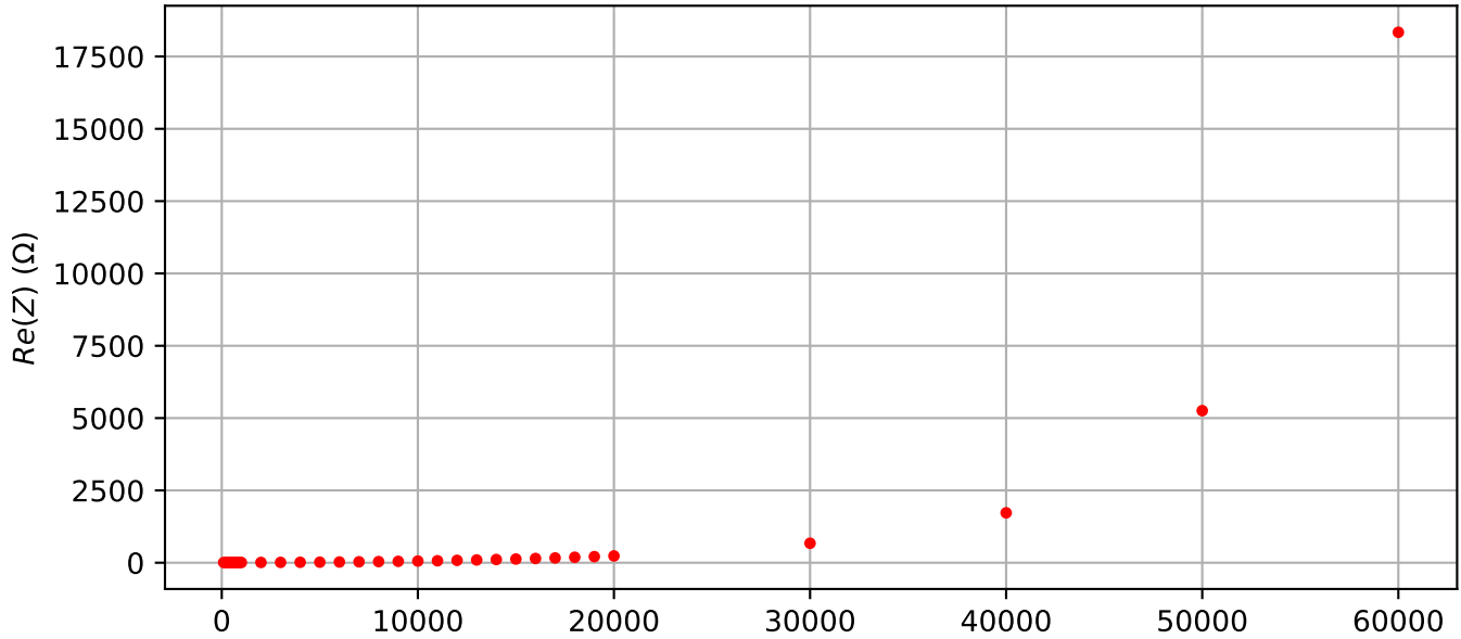
Bobine 2
