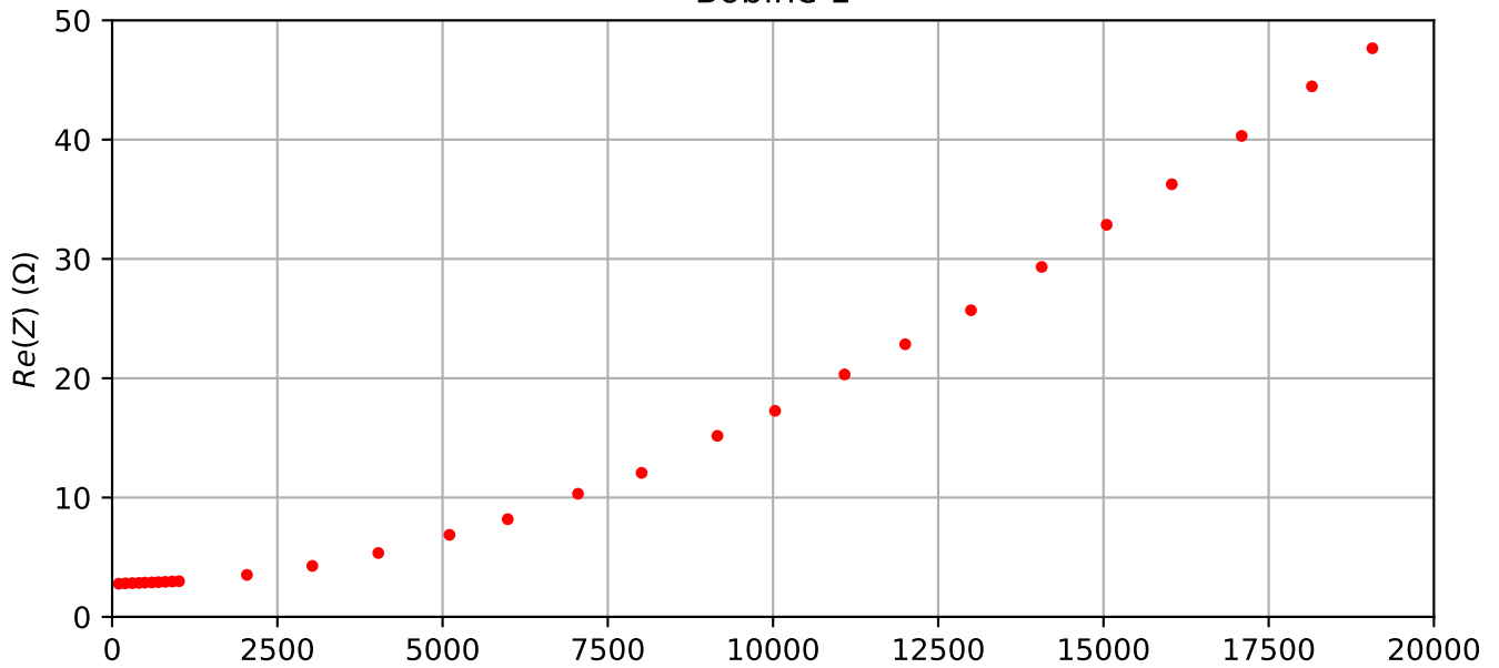
Bobine 1
