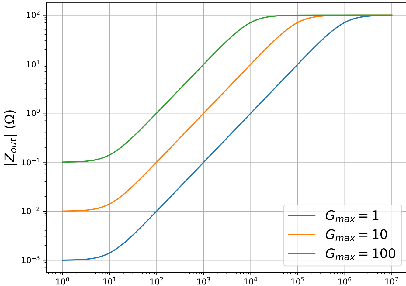
Impédance de sortie pour R_s = 100 Ohms
