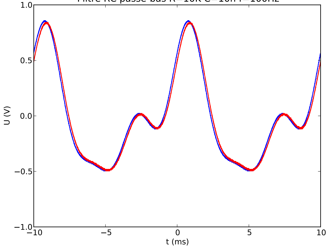
Filtre RC passe-bas R=10K C=10n f=100Hz
