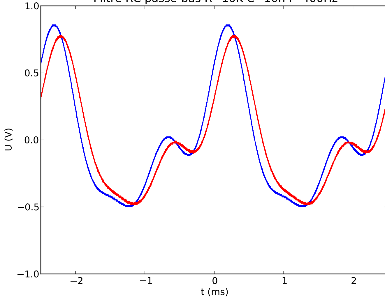
Filtre RC passe-bas R=10K C=10n f=400Hz
